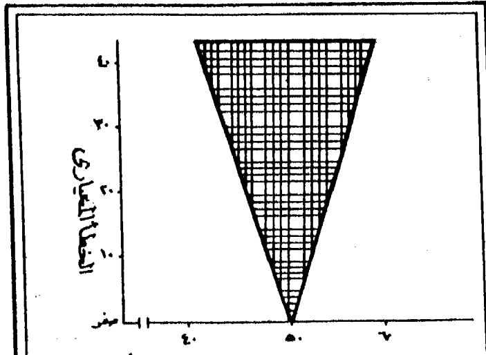
شكل يبين علاقة الانحراف المعياري للعينة وحدود الثقة فيها بنسبة ٩٥٪
